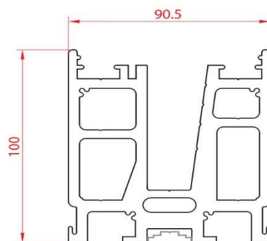
پروفیل شیشه گیر Glass stuck
